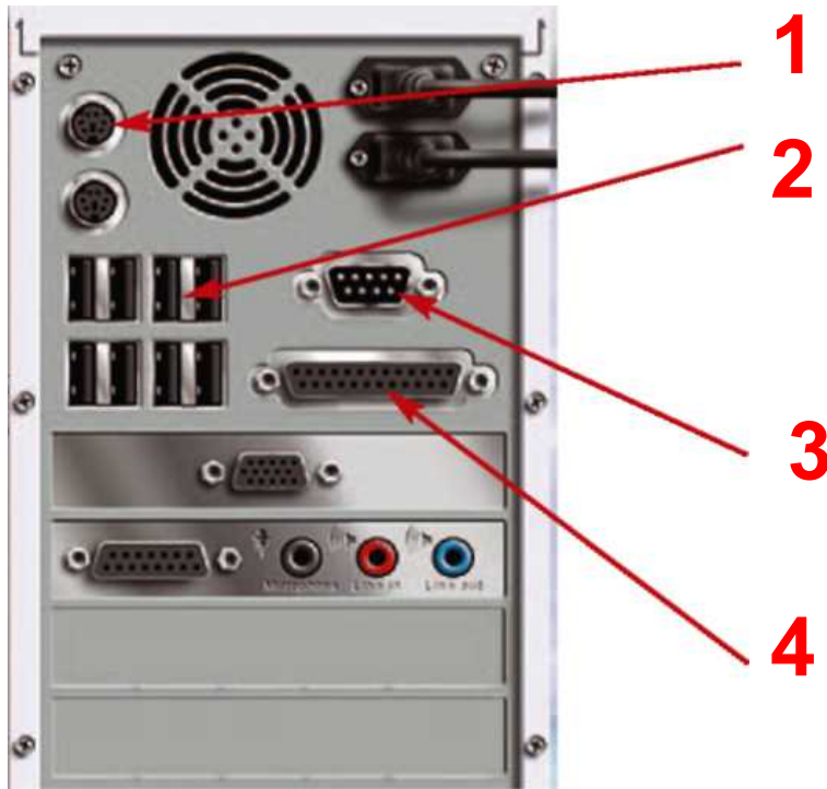
Εικόνα 2.6. Οι θύρες σύνδεσης του υπολογιστή
